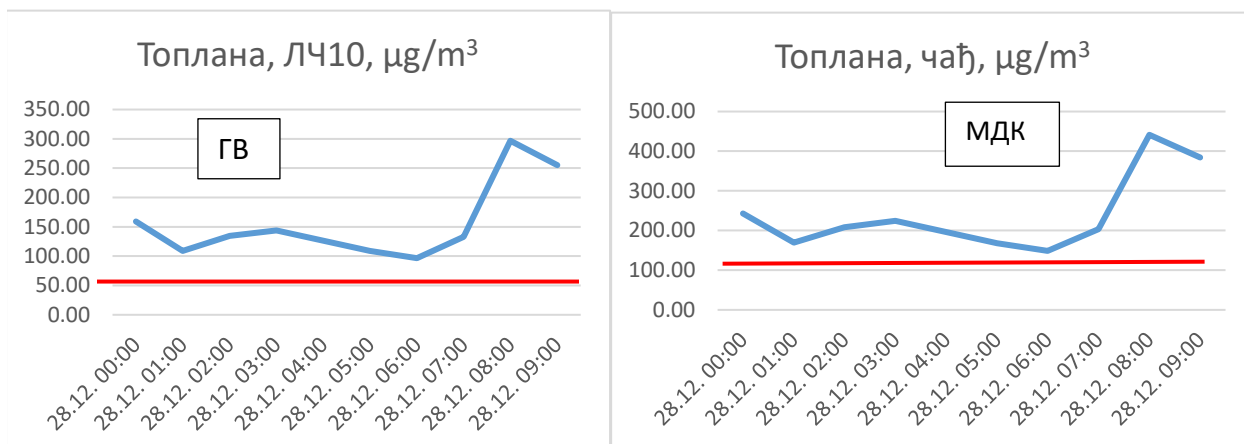
Дијаграми промјена концентрација РМ10 и дима/чађи за првих 9 часова 28.12.2023. године на локацији „Градска топлана“
